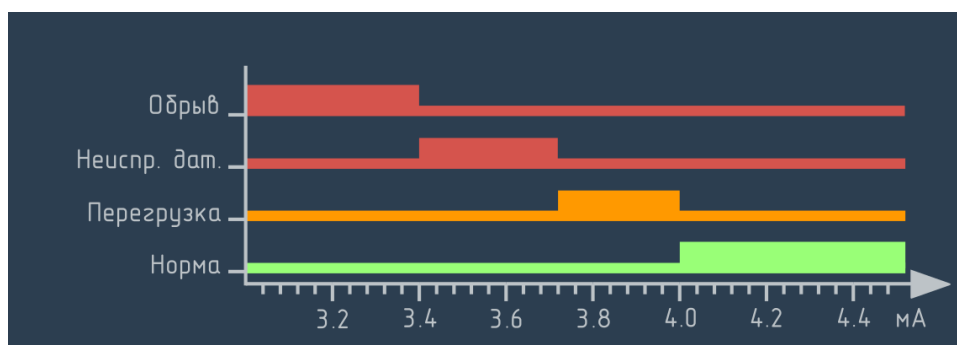
Рисунок 5.3 – Приём сигнала о неисправности датчика, порог срабатывания – меньше 3,75 мА
