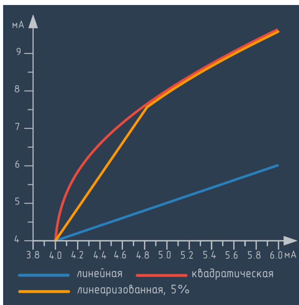
Рисунок 5.12 – Линеаризация передаточной функции «извлечение кв. корня».
