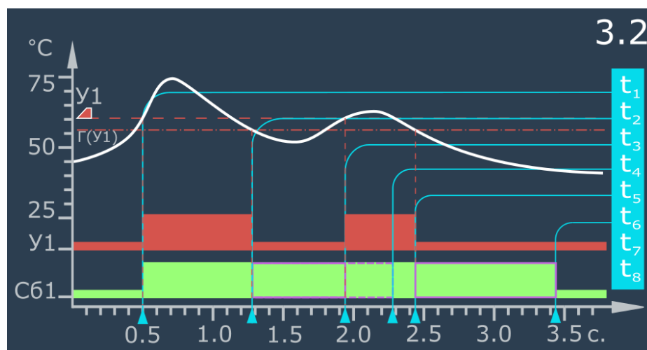
Рисунок 5.23 – Для Сб1 задана длительность по времени 1 с, за время работы таймера длительности происходит повторное срабатывание У1 и У1 остаётся включённой на момент завершения работы таймера длительности.
