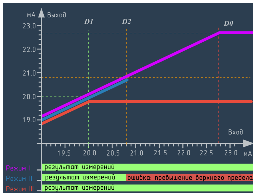
Рисунок 5.6 – режимы обработки выхода за границы назначенного диапазона измерений, масштабируемые сигналы.
