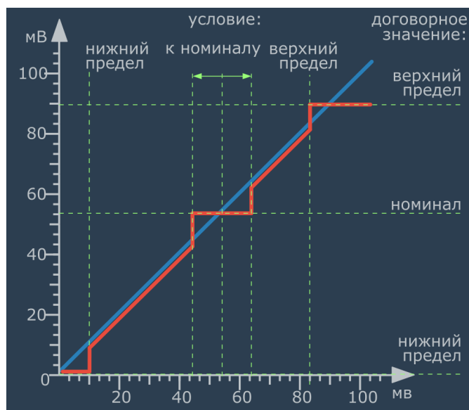
Рисунок 5.13 – работа отсечек.
