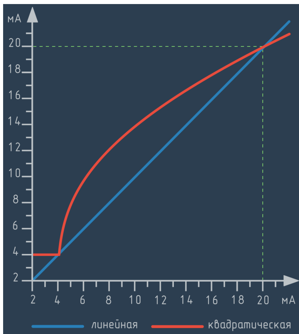
Рисунок 5.11 – график передаточной функции «извлечение кв. корня».
