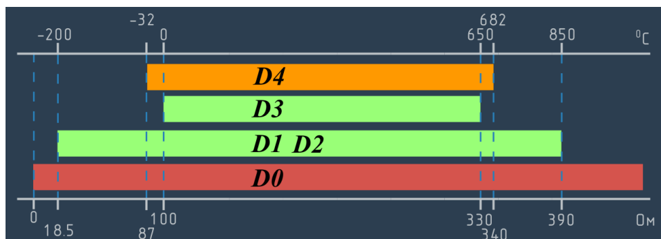
Рисунок 5.5 – Диапазоны измерений аналоговых входов:
