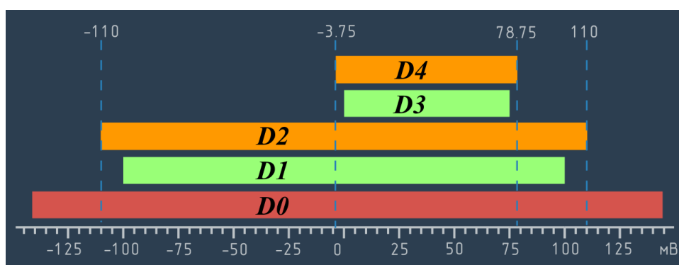
Рисунок 5.4 – Диапазоны измерений аналоговых входов:
