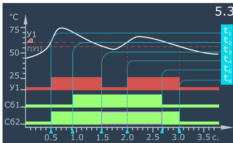
Рисунок 5.29 – Для Сб1 задана "длительность", режим "по событию" Сб2, условия для срабатывания Сб1 восстанавливаются в то время, когда Сб2 находится в состоянии «1».
