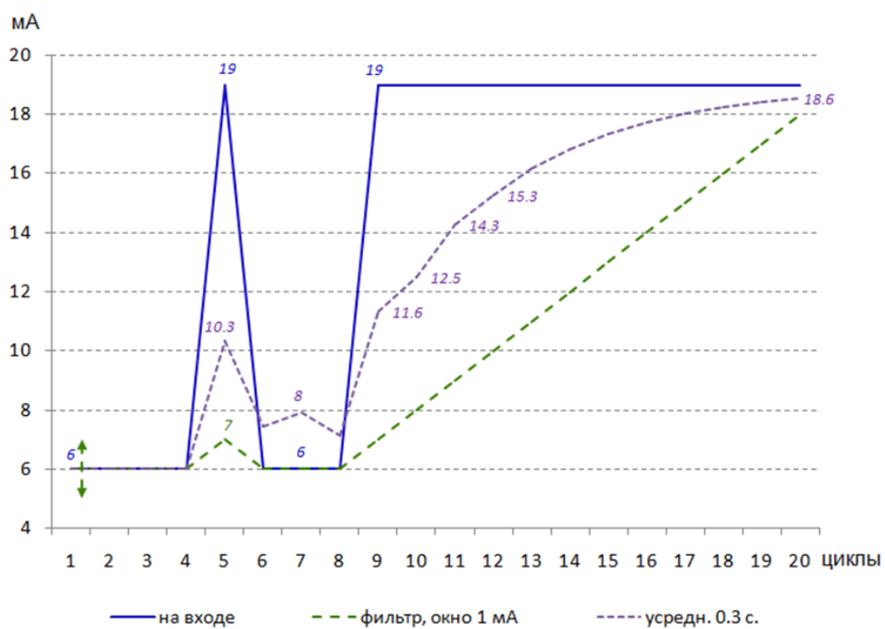
Рисунок 5.9 – вычисление скользящего среднего.
