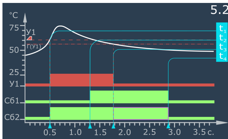
Рисунок 5.28 – Для Сб1 задана "длительность", режим "по событию" Сб2, Сб1 срабатывает, когда Сб2 в состоянии «0».
