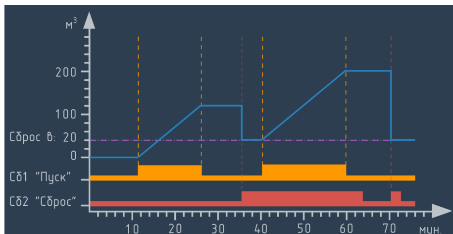
Рисунок 6.45 – График работы счётчика. "Вычисление" – "Сб1", "Сброс" – "Сб2"
