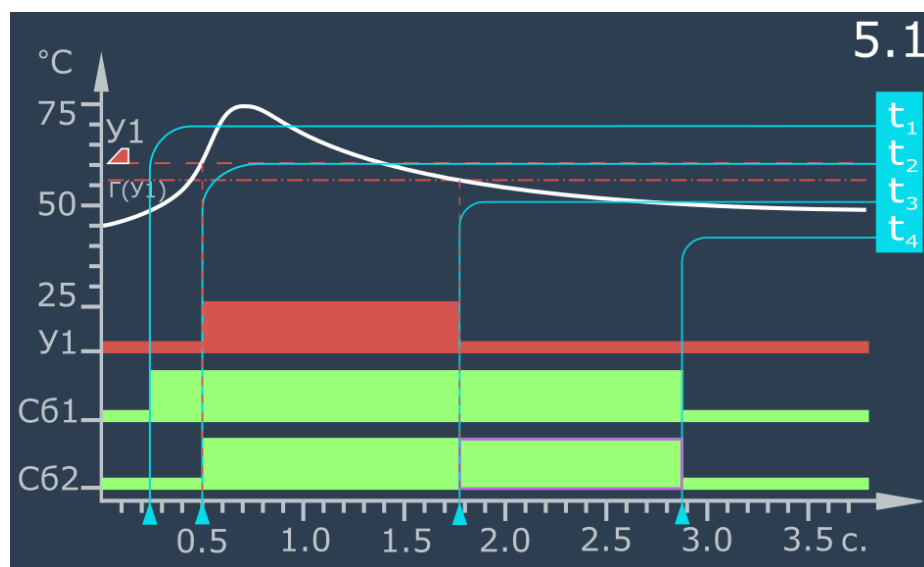
Рисунок 5.27 – Для Сб1 задана "длительность", режим "по событию" Сб2, Сб1 срабатывает, когда Сб2 в состоянии «1».
