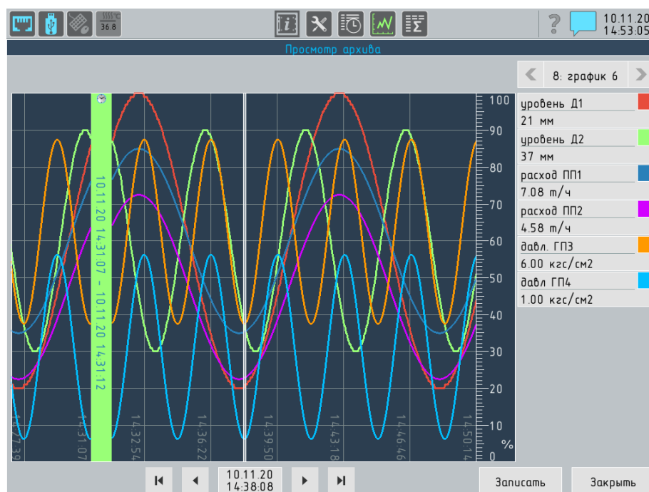
Рисунок 4.23 – Режим "Архив"
