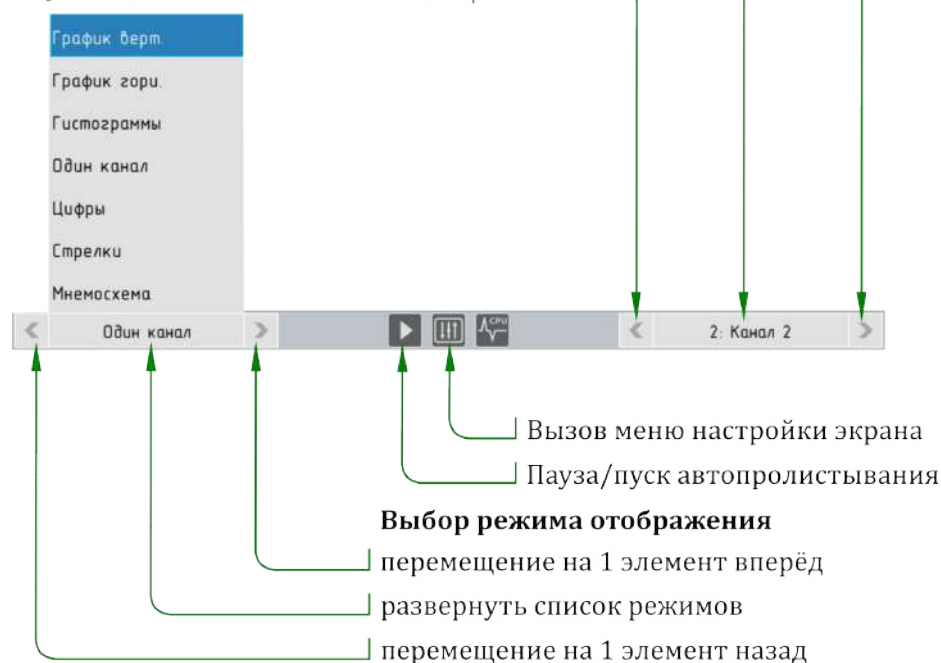
Рисунок 3.7 – панель навигации
