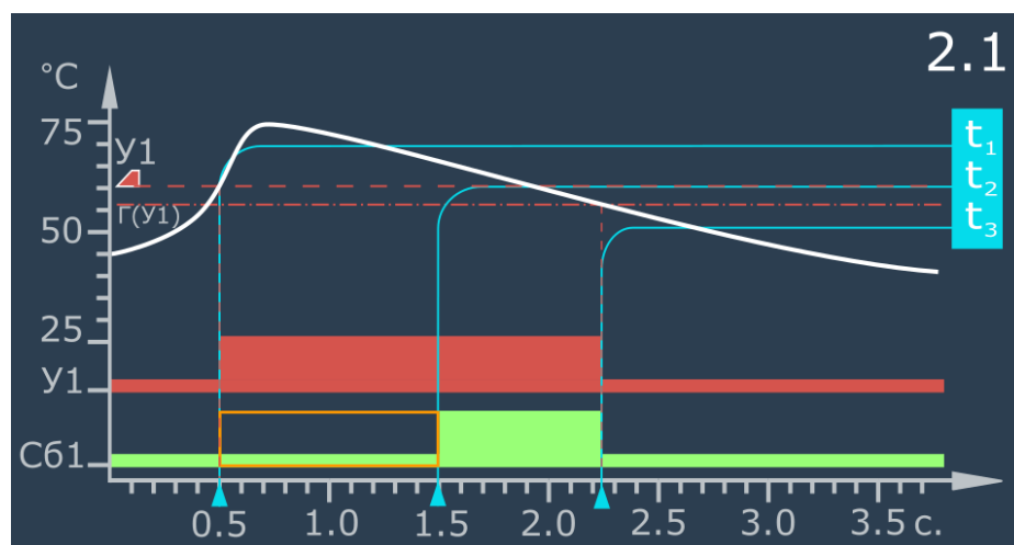
Рисунок 5.19 – Для Сб1 задана задержка срабатывания 1 с, время, в течение которого уставка была превышена, больше, чем величина задержки.
