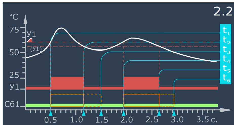
Рисунок 5.20 – Для Сб1 задана задержка 1 с, время, в течение которого уставка была превышена, меньше, чем величина задержки.
