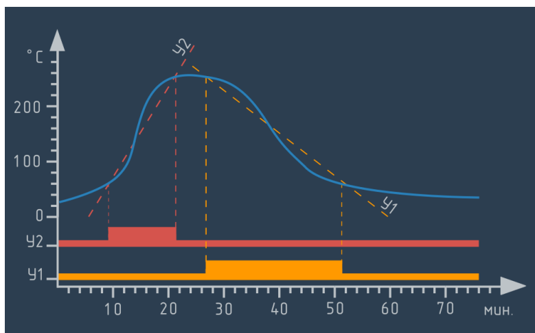
Рисунок 5.15 – Работа уставок, аргумент – скорость изменения результата измерений: U1 тип «больше», значение уставки > 10\text{ }^{\circ}\text{C}/\text{мин} , гистерезис не назначен; U2 тип «меньше», значение уставки < 5\text{ }^{\circ}\text{C}/\text{мин} , гистерезис не назначен.
