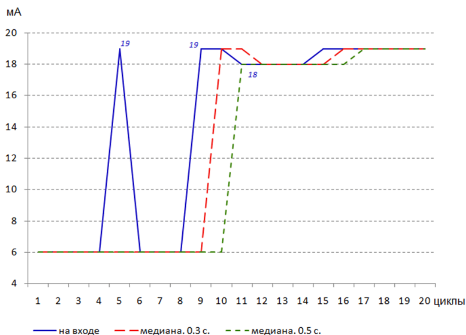
Рисунок 5.10 – вычисление скользящего среднего.
