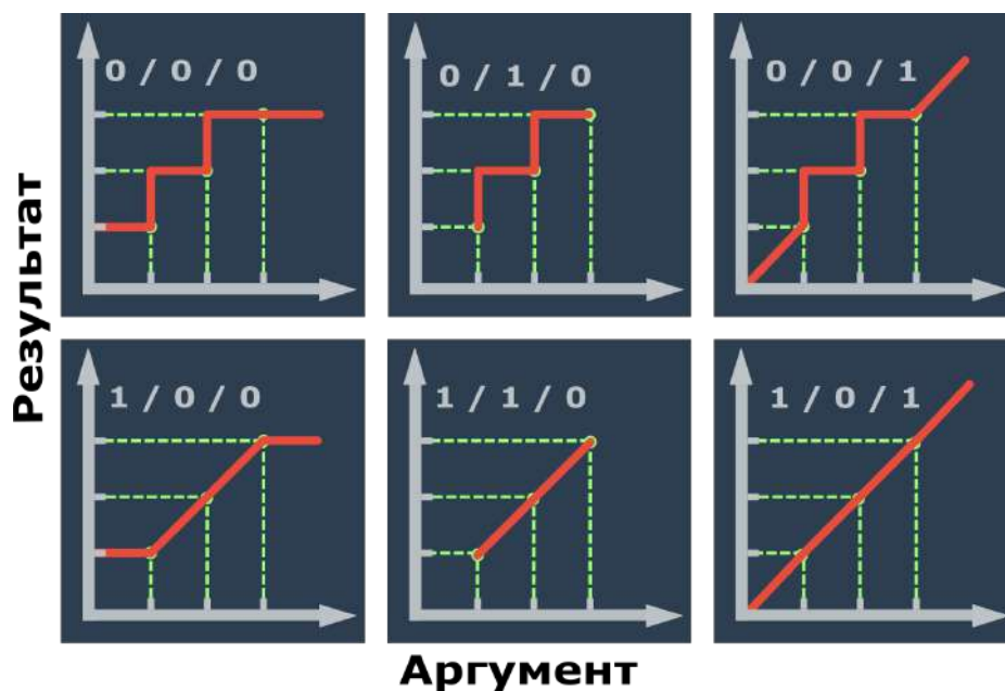
Рисунок 6.39 – График функции, заданной с помощью таблицы состояния флагов (0/1): "Интерп." / "Строго" / "Экстрап."
