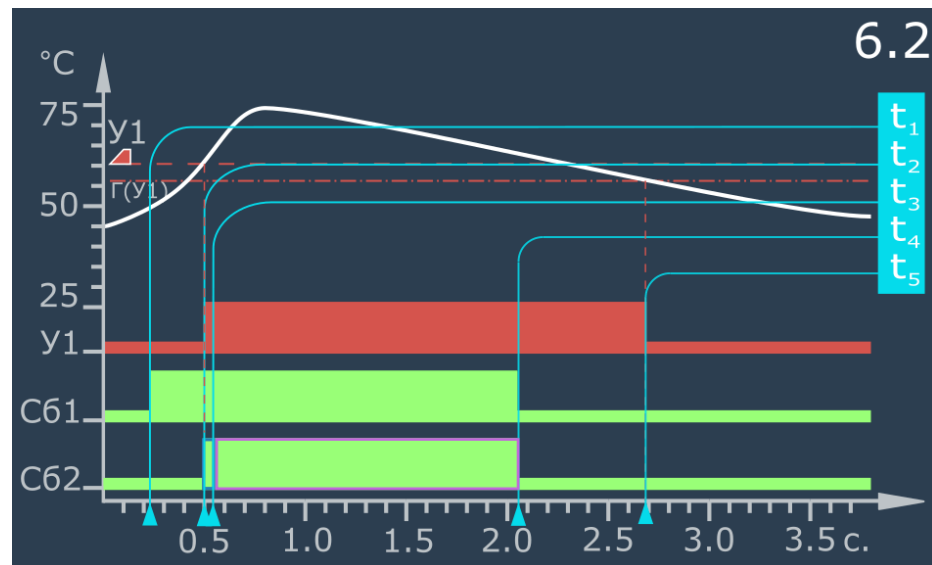
Рисунок 5.31 – Для Сб1 задан признак "однократное" и длительность "по событию" Сб2, в момент отключения Сб2 условие на срабатывание Сб1 выполняются.
