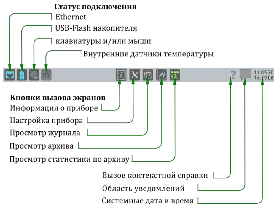
Рисунок 3.5 – Панель задач
