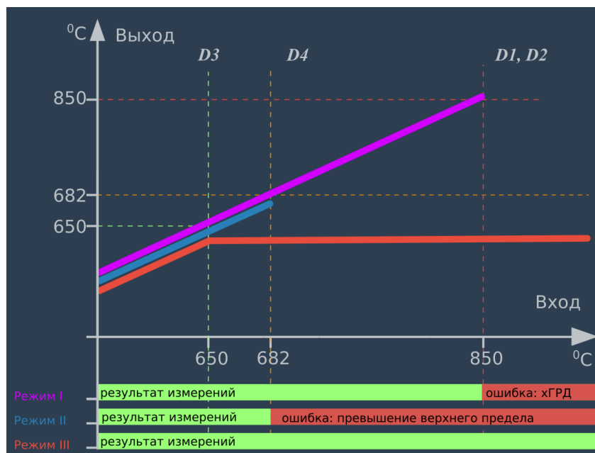
Рисунок 5.7 – режимы обработки выхода за границы назначенного диапазона измерений, немасштабируемые сигналы.
