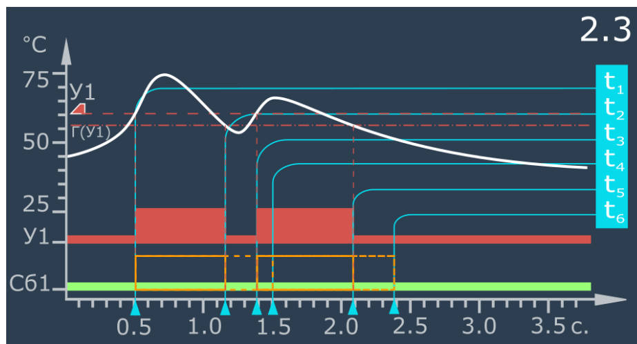
Рисунок 5.21 – Для Сб1 задана задержка 1 с, время, в течение которого уставка была превышена, меньше, чем величина задержки, при этом повторное срабатывание уставки происходит до истечения времени задержки, заданного первым срабатыванием.
