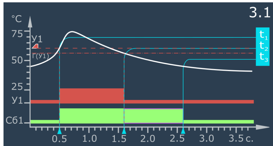
Рисунок 5.22 – Для Сб1 задана длительность "по времени" 1 с.
