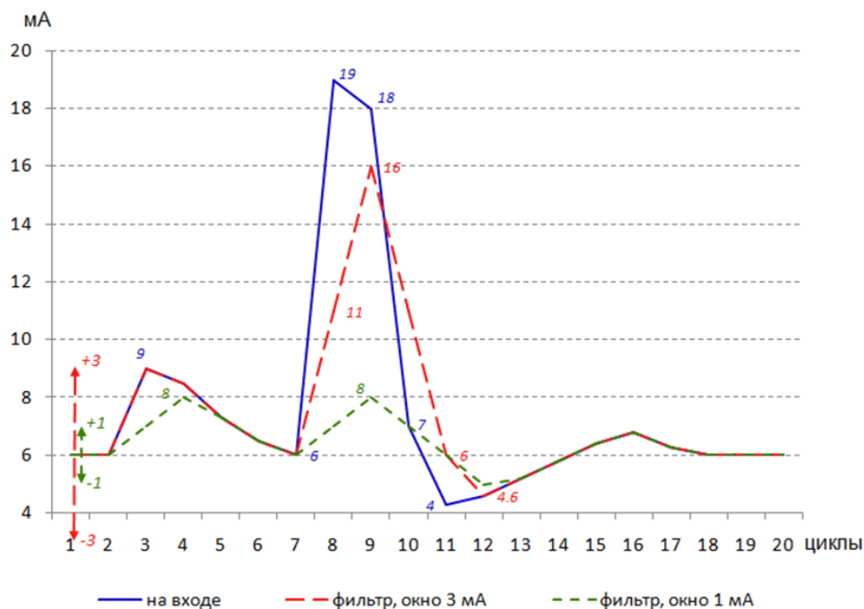
Рисунок 5.8 – вычисление скользящего среднего.
