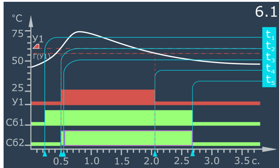
Рисунок 5.30 – Для Сб1 задан признак "однократное" и "длительность", режим "по событию" Сб2, в момент отключения Сб2 условие на срабатывание Сб1 выполняются.
