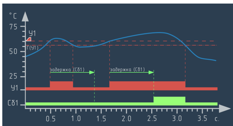
Рисунок 6.80 – График работы задержки срабатывания события. Для С1 установлена задержка 0.8 с.
