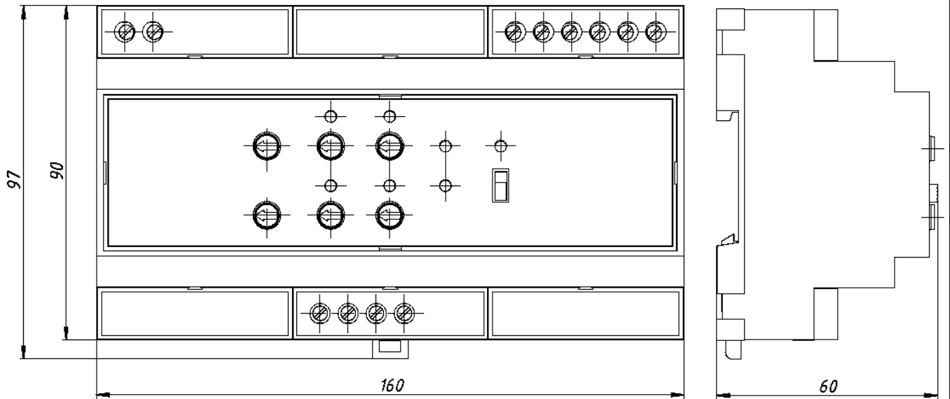
Рисунок А.1 – Габаритные размеры РЗН-1001
