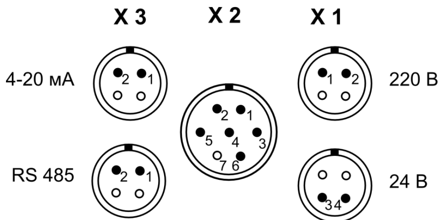
Рисунок 8 – Распайка контактов разъёмов прибора Ф1791.2
