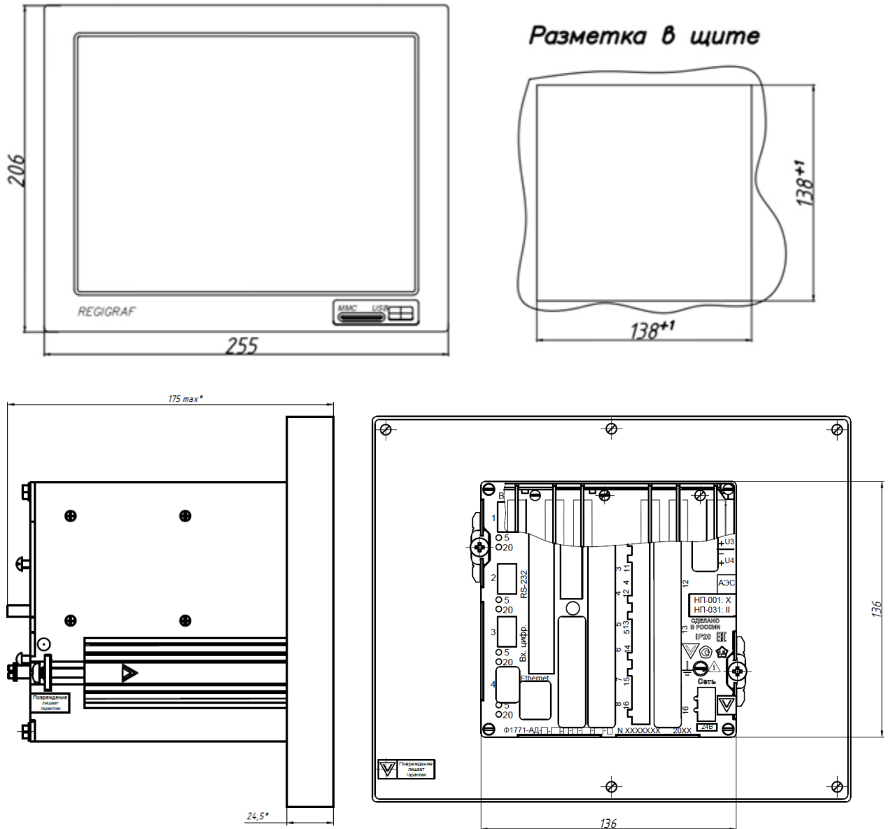
Рисунок 1 – Габаритный чертёж прибора и вырез в щите
