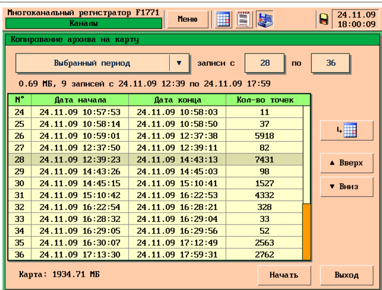
Рисунок 22 – Копирование архива на Flash-накопитель
