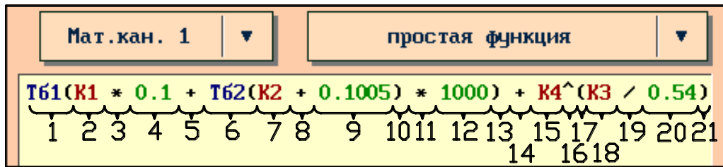
Рисунок 48 – Пример подсчета числа аргументов и операторов МК
