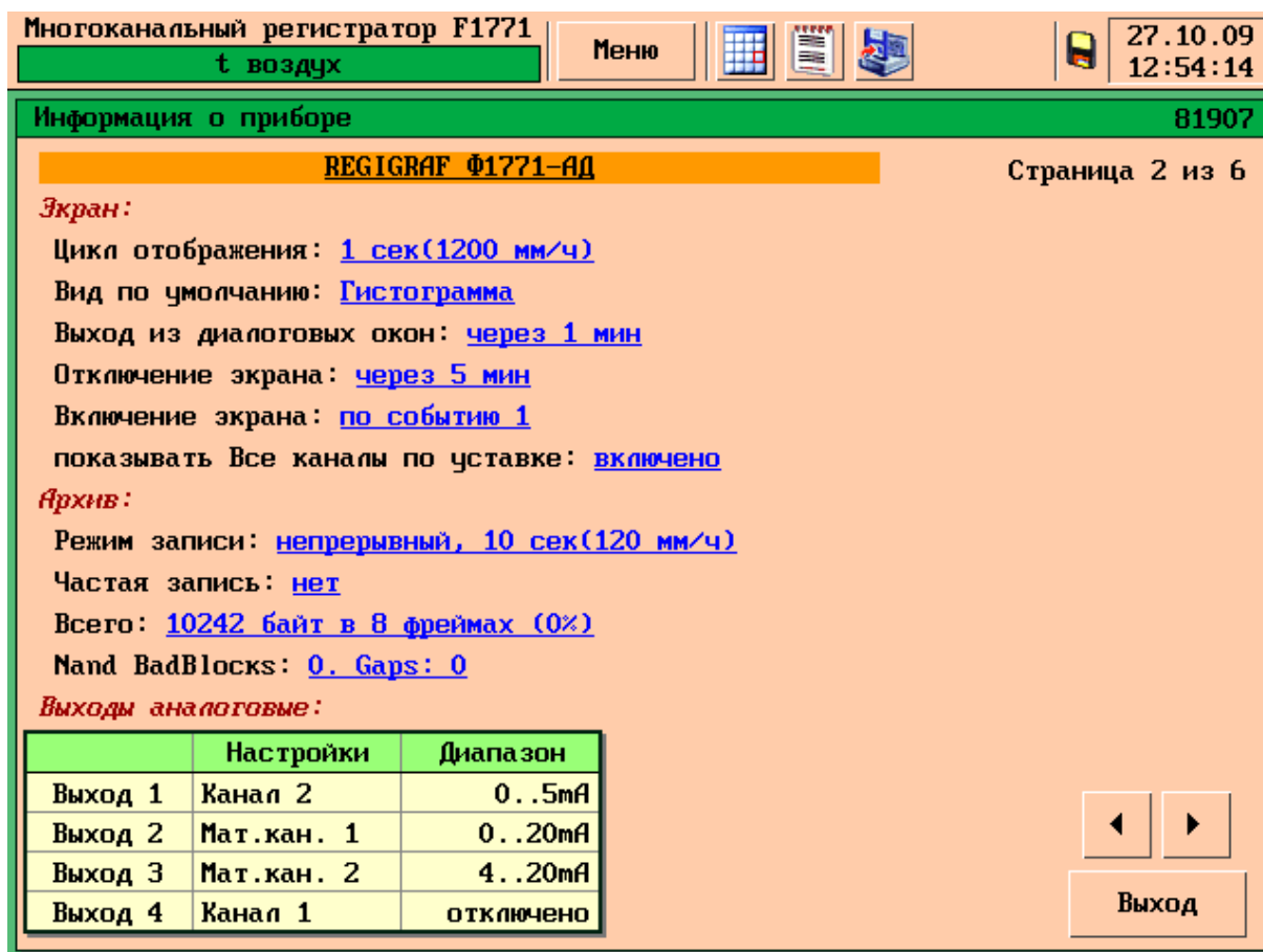
Рисунок 6 – Информация о приборе страница 2: настройки экрана, архива и аналоговых выходов
