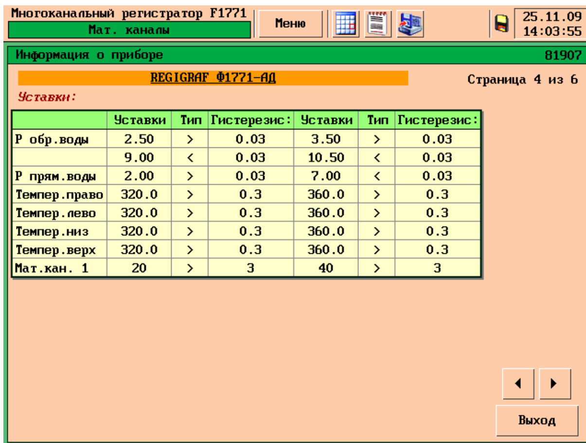
Рисунок 8 – Информация о приборе страница 4: настройки уставок
