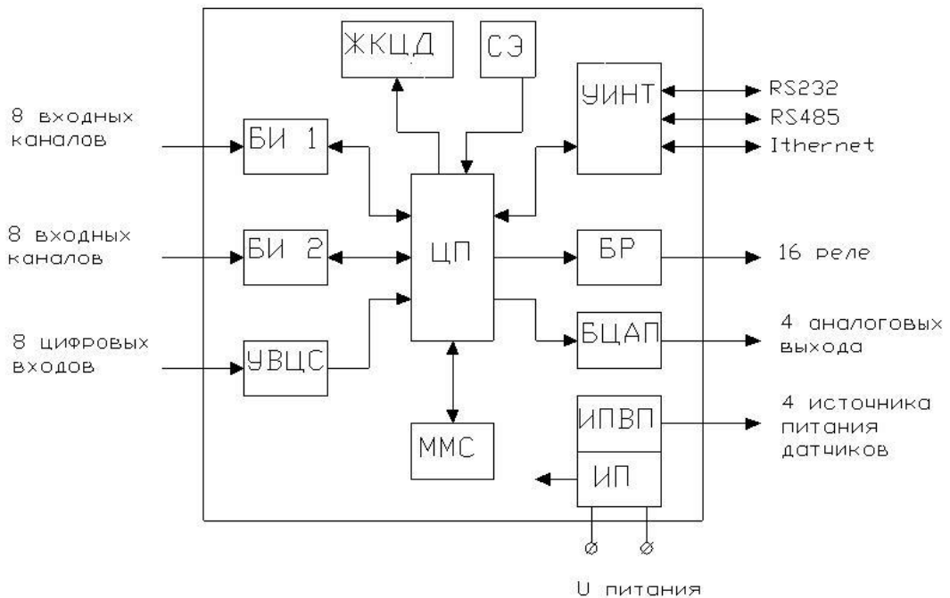
Рисунок 2 – Функциональная схема прибора
