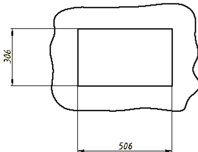
Рисунок А.4 – вырез в щите для видеомонитора в исполнении ВМП1225-АД-5-Х-Х-1 (для установки в панельный щит)
