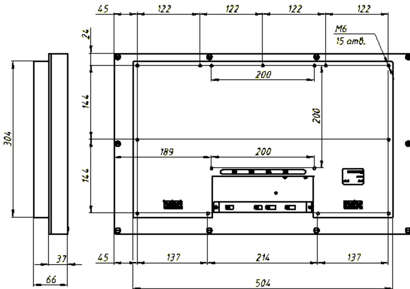
Рисунок А.2 – Габаритный чертёж видеомонитора в исполнении ВМП1225-АД-5-Х-Х-Х, вид сбоку и сзади, положения отверстий для крепления в щите и крепления VESA
