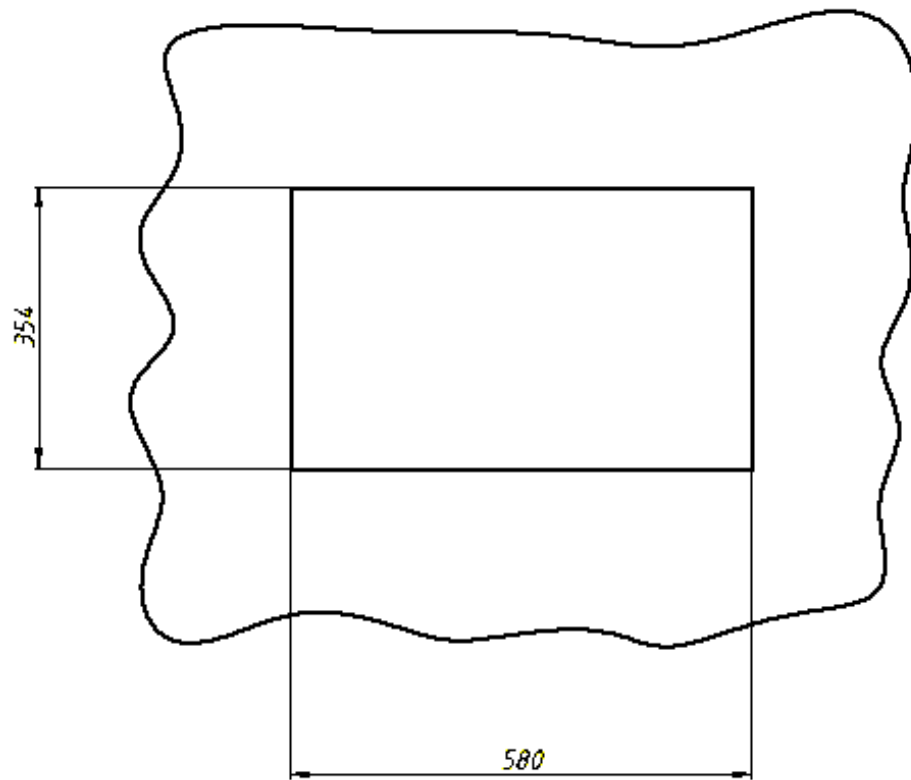
Рисунок А.3 – вырез в щите для видеомонитора в исполнении ВМП1225-АД-5-Х-Х-2 (для установки в мозаичный щит)
