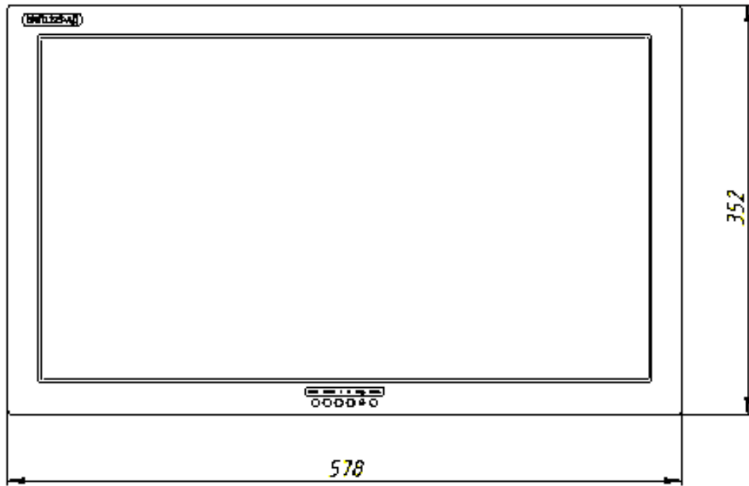
Рисунок А.1 – Габаритный чертёж лицевой части видеомонитора в исполнении ВМП1225-АД-5-Х-Х-Х
