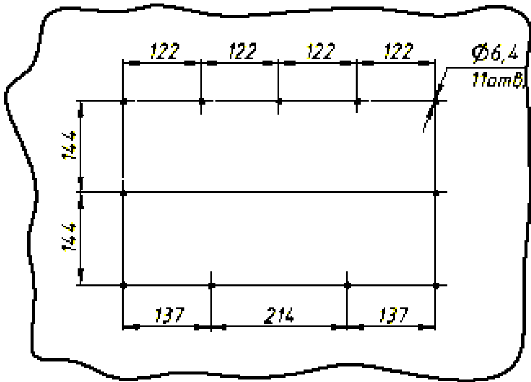
Рисунок А.6 – расположение отверстий в пластине для крепления видеомонитора в исполнении ВМП1225-АД-5-Х-Х-2 в мозаичный щит.
