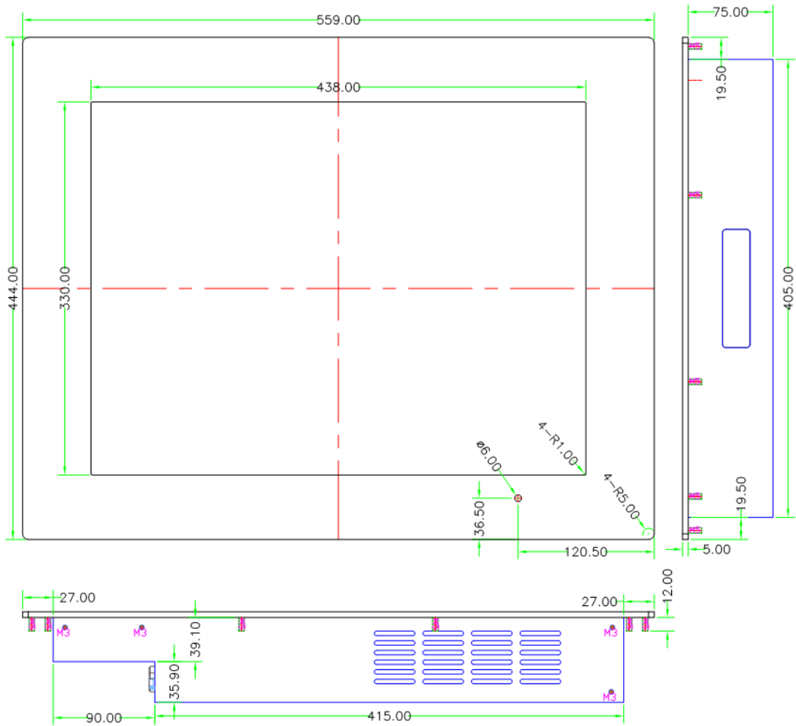
Рисунок А.7 – Габаритный чертёж видеомонитора в исполнении ВМП1225-АД-8-Х-Х-Х.
